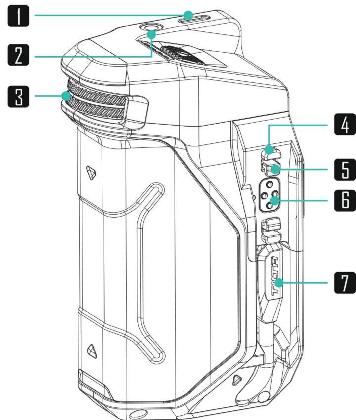
&lt;正面&gt;
