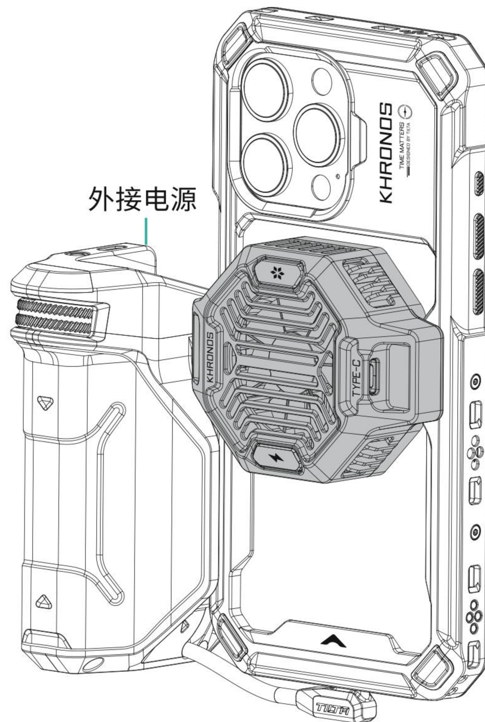
&lt; 带手机壳状态 &gt;
